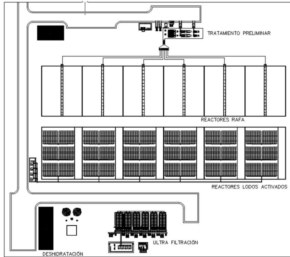
Imagen No. 28. Planta de Tratamiento de Punta Cana
