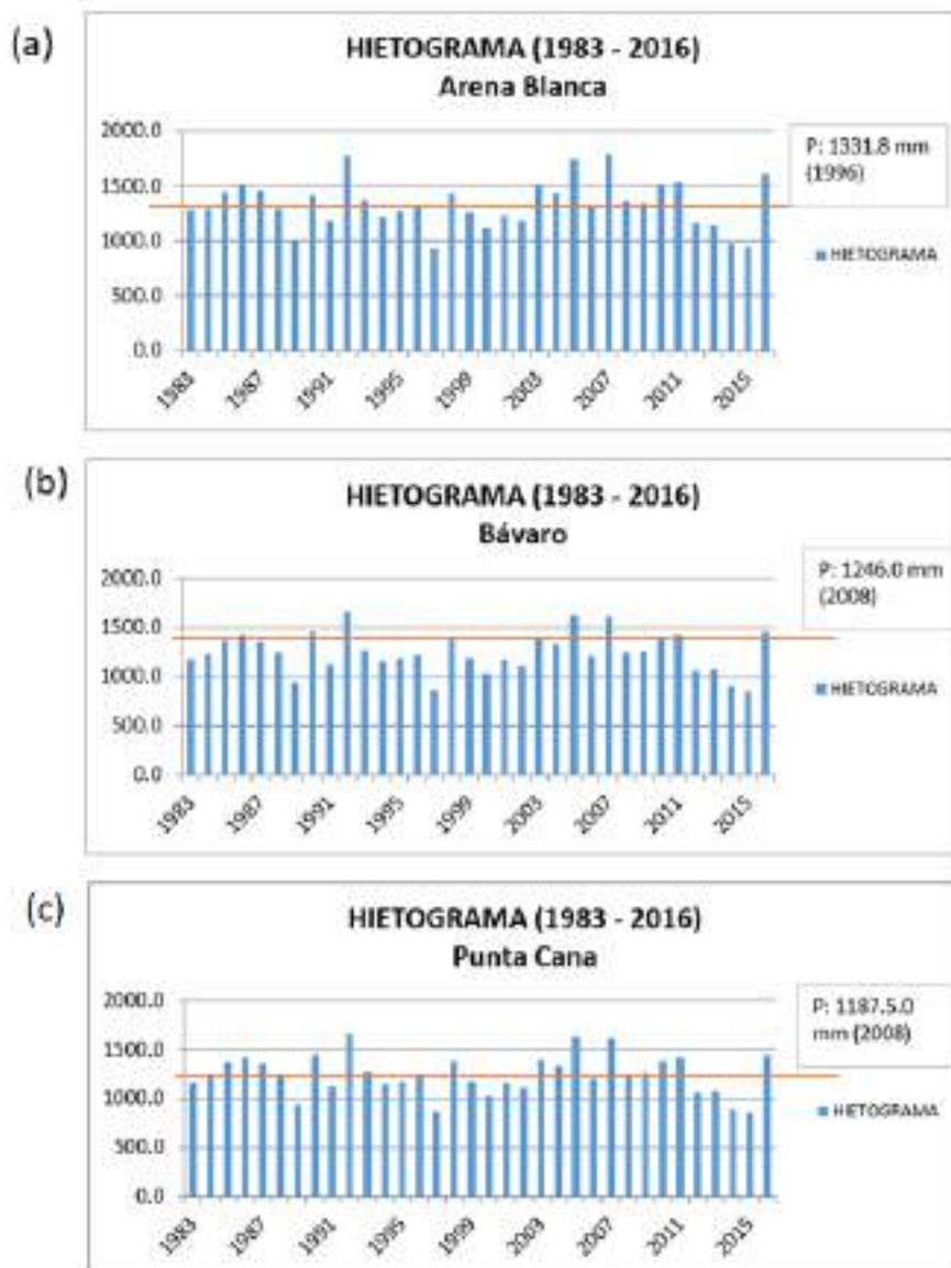
Imagen No. 33. Precipitación media de un “Año normal” de las 3 sub-zonas de extracción del acuífero en situación actual. Fuente.: (Equipo de Consultores Externos del Banco Interamericano de Desarrollo, 2025)
