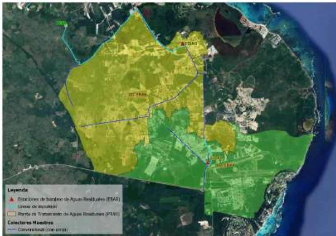
Imagen No. 15. Sistema proyectado para Verón
