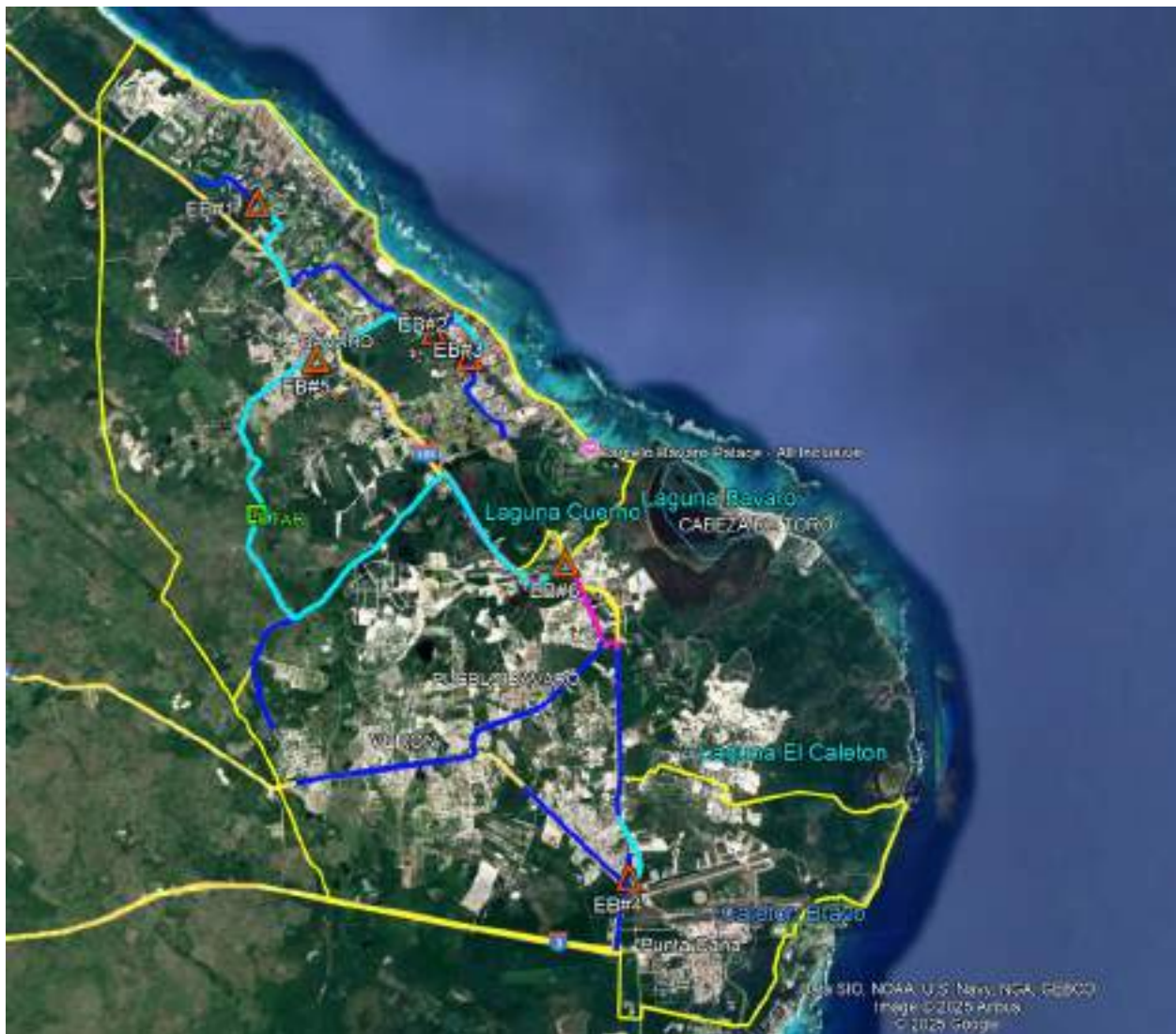
Imagen No. 37. Macro estructura del alcantarillado sanitario regional de Punta Cana - Bávaro
