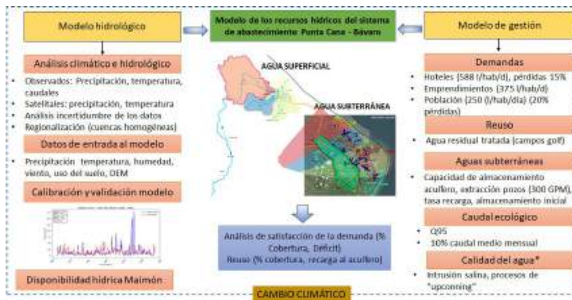
Imagen No. 34. Esquema de construcción del modelo hidrológico y de gestión del sistema de abastecimiento de agua potable Verón - Punta Cana
