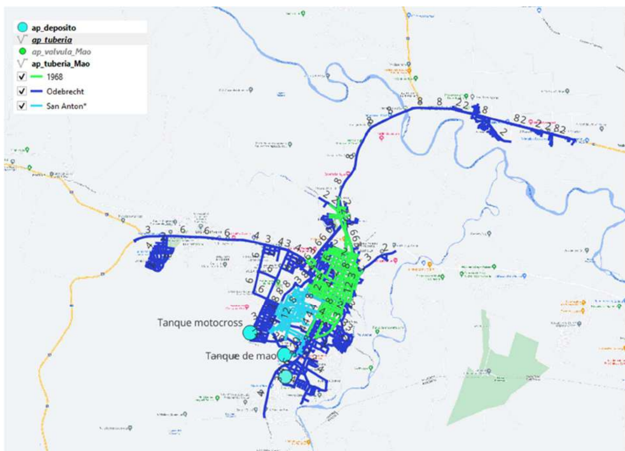
Figura: Plano general del sistema ALINO
