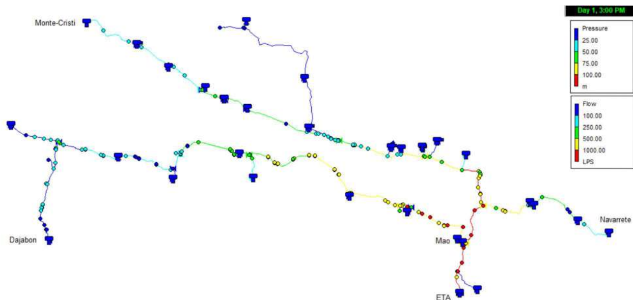
Figura: Resultados de la modelización de día del sistema ALINO al momento del diagnóstico detallado de la AT - Noviembre 2022 (Fuente: SEURECA).
