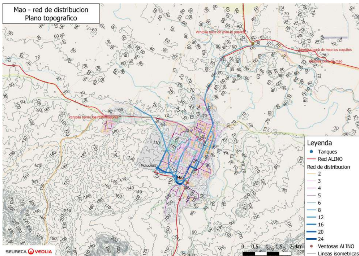
Plano de la topografía en Mao (Fuente: SIG preparado por SEURECA con la información de los planos comunicados por el INAPA)
