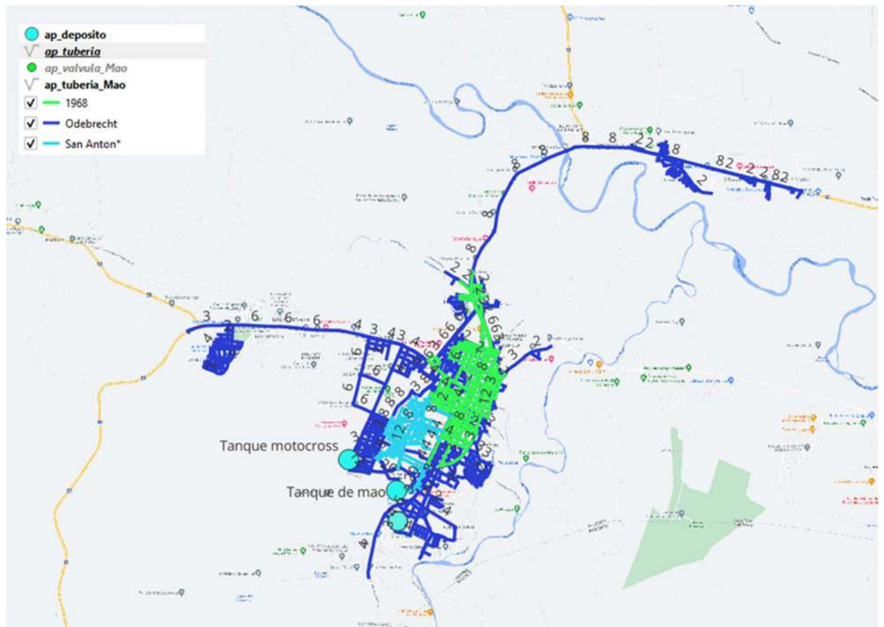
Figura: Plano general del sistema ALINO (Fuente: SIG preparado por SEURECA con la información de los planos comunicados por el INAPA)
