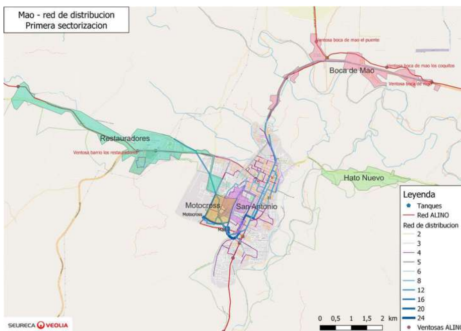
Primera propuesta de sectorización del sistema hidráulico de Mao
